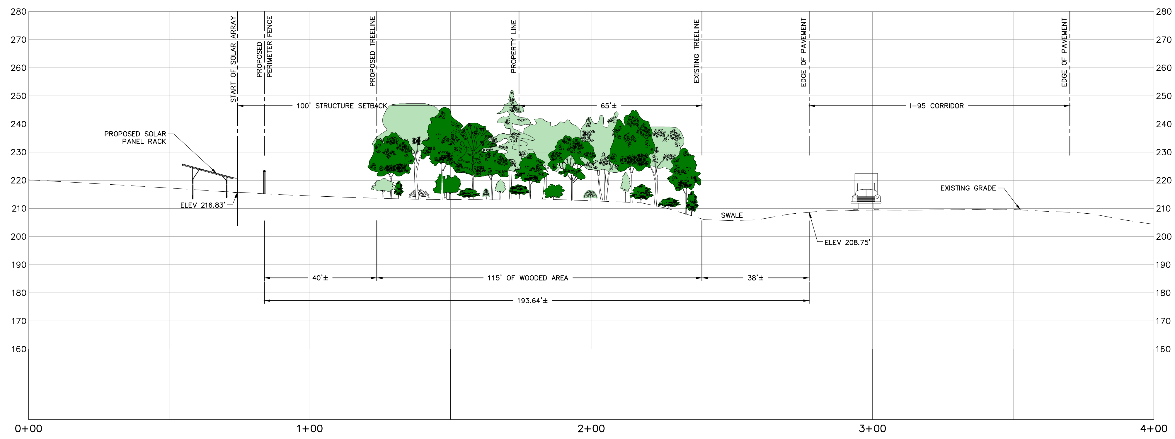
PROFILE STA. 0+00 TO STA. 4+00 HORIZONTAL SCALE: 1" = 20' VERTICAL SCALE: 1" = 20'
